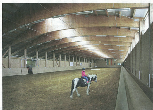
Die Eibenstocker Reithalle ist nach Angaben des Betreibers die wahrscheinlich längste, in Holzbinderbauweise gefertigte Reithalle Deutschlands. Sie ist allerdings nicht für Turniere ausgelegt, sondern widmet sich vorrangig dem Jugend- und Breitensport. BILDER (3): LARS ROSENKRANZ
